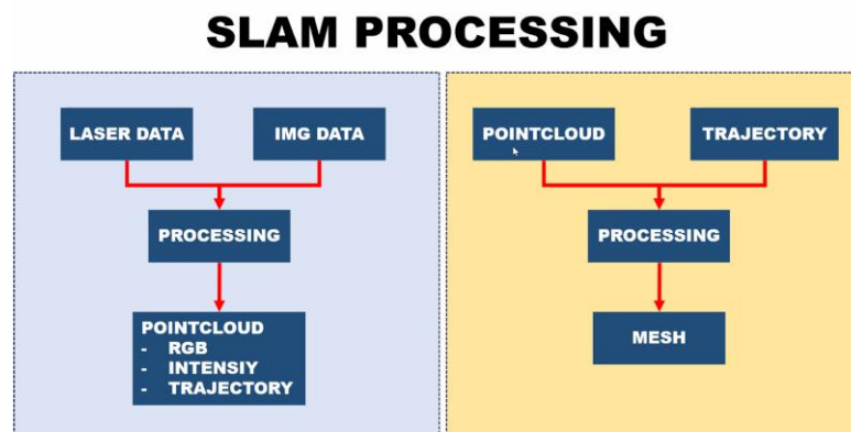
รูปที่ 6 กระบวนการทำงานของ SLAM โดยรวม
