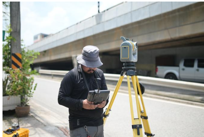
รูปที่ 24 การใช้ LiDAR Scanner เก็บข้อมูลพิกัด
