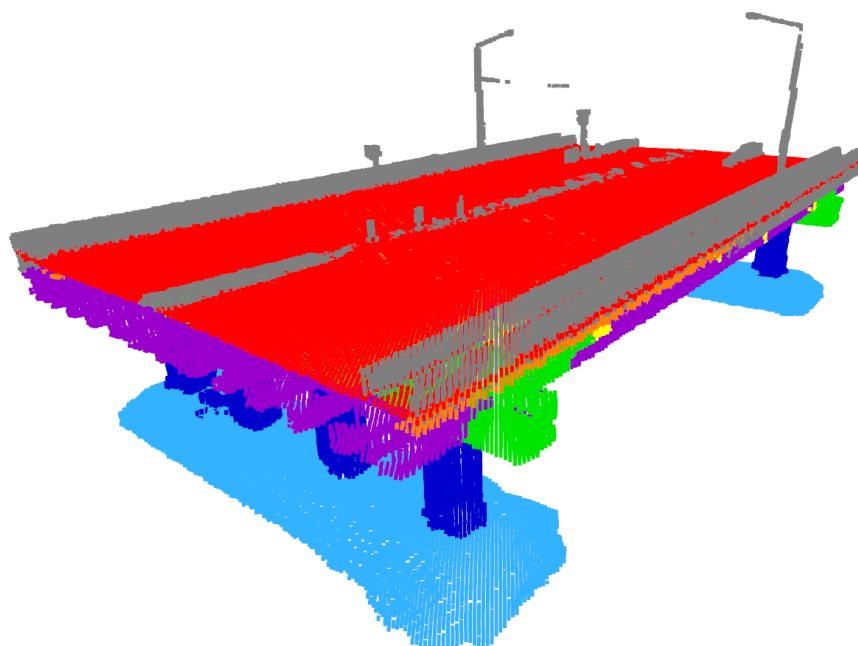
รูปที่ 25 การจำแนกองค์ประกอบของสะพานแบบอัตโนมัติ
