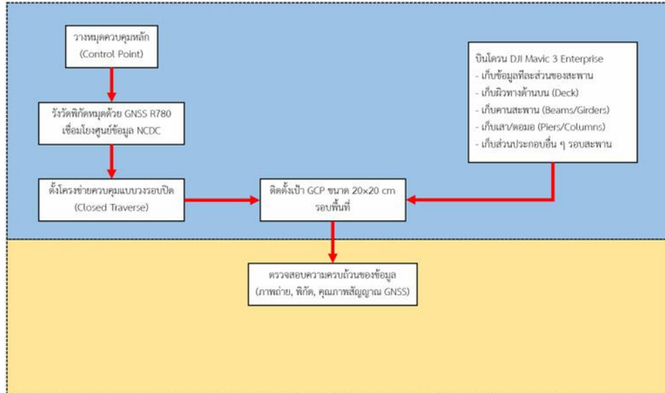
รูปที่ 19 ขั้นตอนการเตรียมการและการเก็บข้อมูลภาคสนาม
