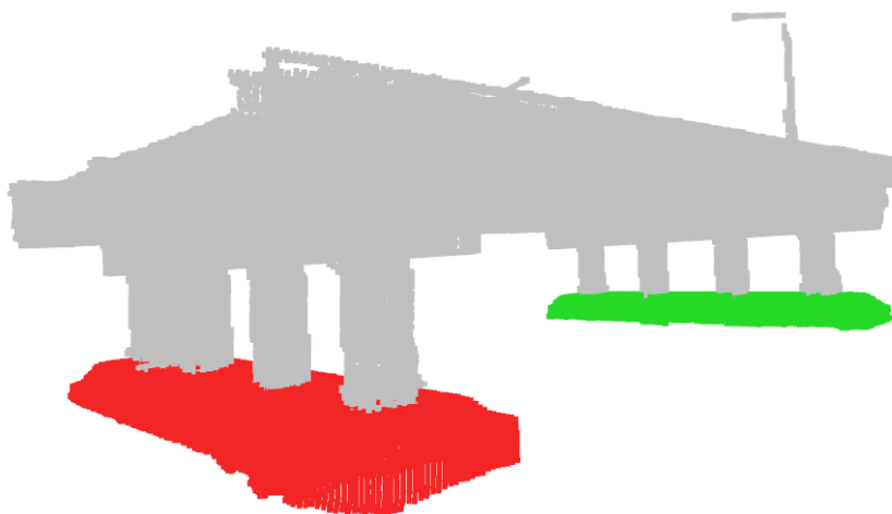
รูปที่ 28 การจัดกลุ่มของ Lower Pier Cap
