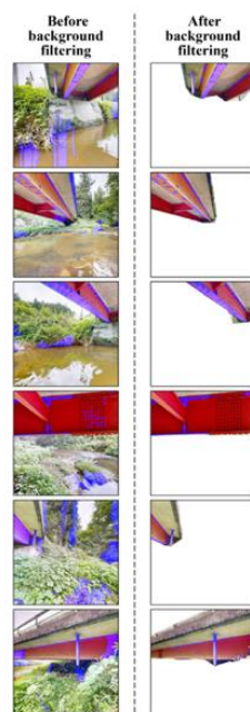
รูปที่ 8 ภาพเปรียบเทียบการตรวจจับการกัดกร่อนก่อนและหลังการใช้พอยต์คลาวด์ 3 มิติเพื่อกรองพื้นหลัง (Lin et al. , 2025)
