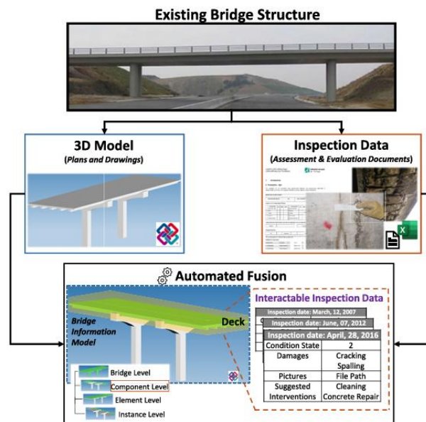
รูปที่ 9 แผนภาพการทำงานของ การผสานข้อมูลจาก 3D Model, BMS.DB เข้าด้วยกันเป็น BrIM Model (Santos et al. , 2025)
