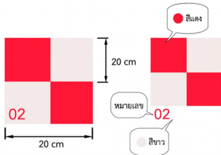
รูปที่ 13 Ground Control Point – GCP Target Sticker
