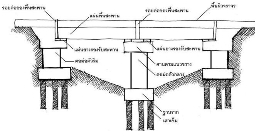
รูปที่ 2 องค์ประกอบของโครงสร้างสะพาน
