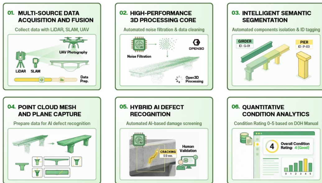
รูปที่ 16 กระบวนการวิจัยสำหรับประเมินสภาพสะพาน
